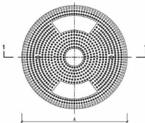
平面图
