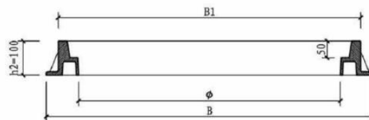
1-1剖面图
