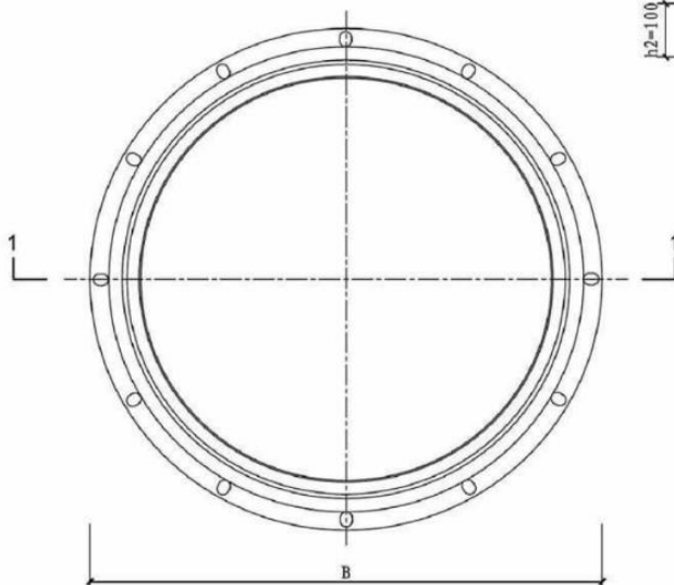
平面图
