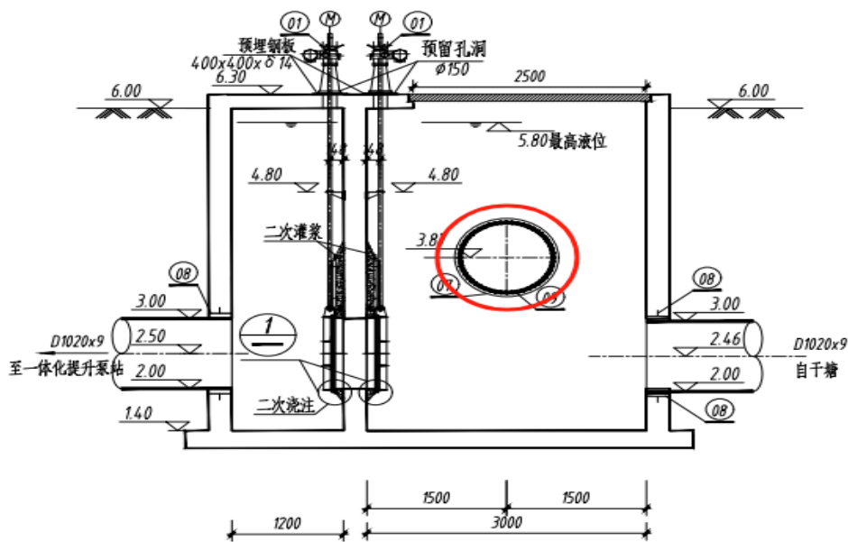
1号闸门井A-A剖面图 1:50
