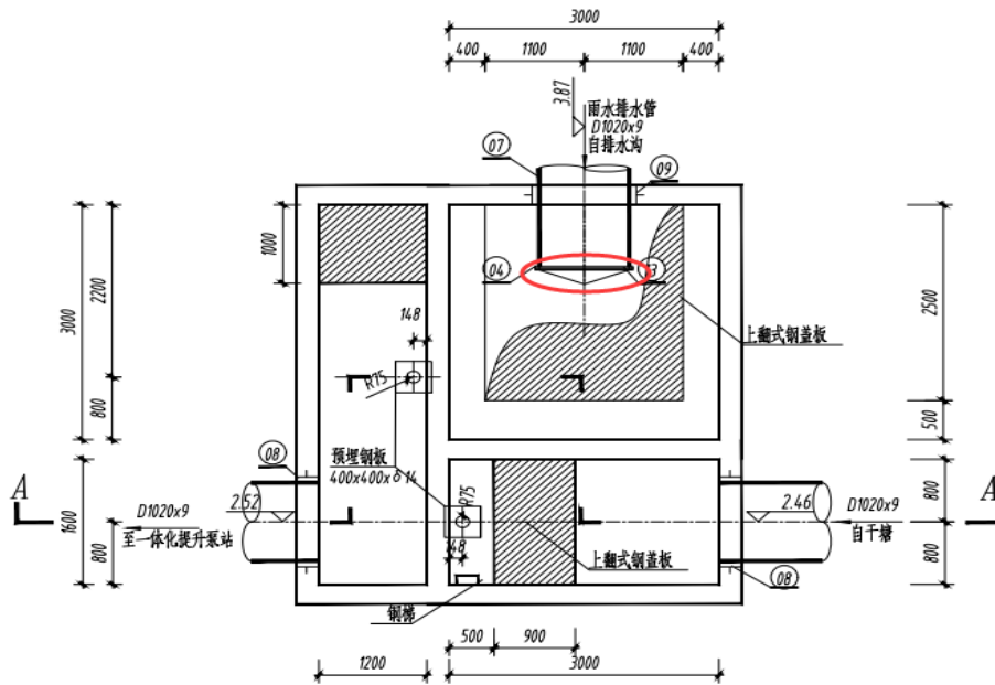
1号阀门井平面图 1:50
