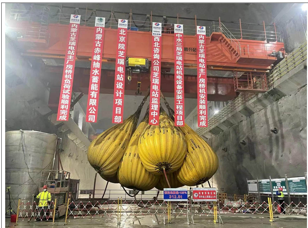
图 1: 水袋负荷试验示意图
