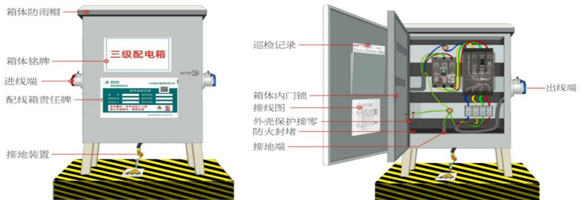
图 91 传统三级施工电源柜示例图
