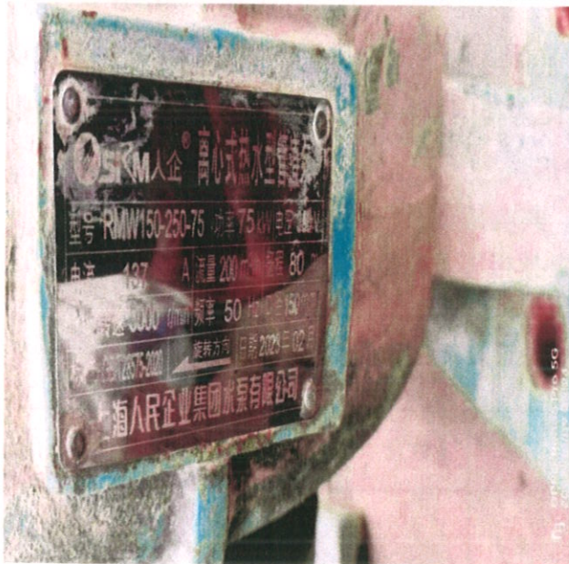
水泵名牌
