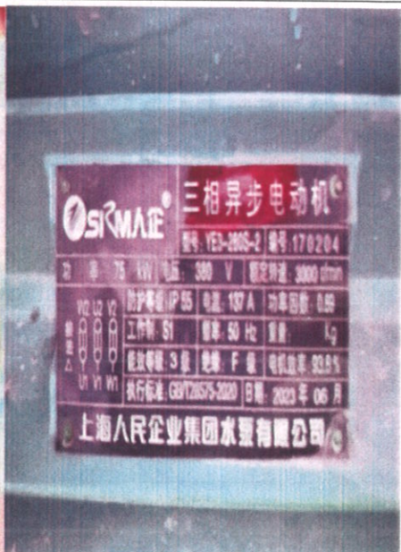
电机名牌
